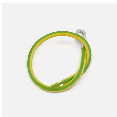
MK-10-GG-60 MK 10 gulgrön kabel med kabelsko CU/AL 60 cm
